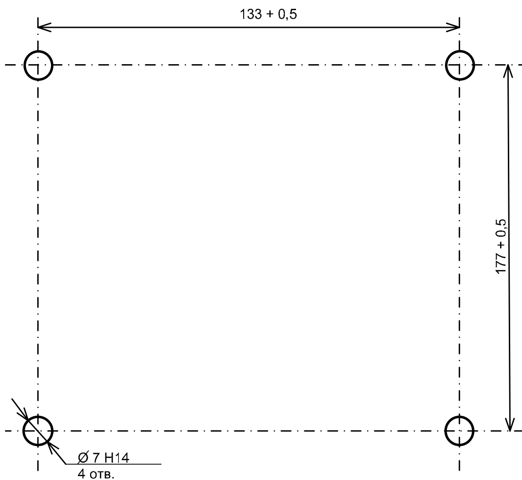
Рисунок 2 – Разметка щита для крепления блока
