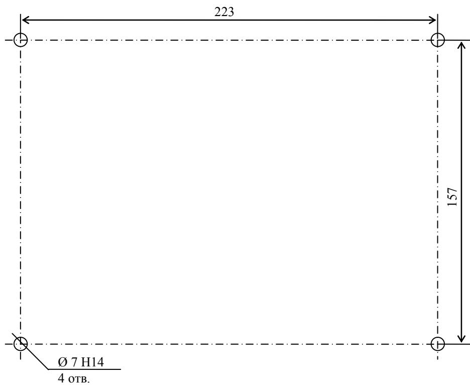
Рисунок 3 – Разметка щита для крепления прибора
