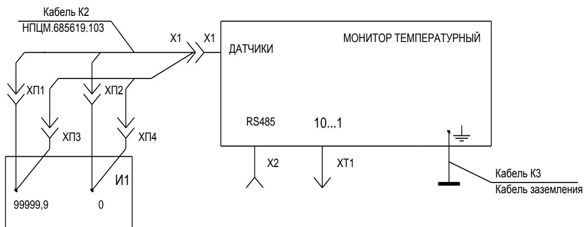
Рисунок 5 – Схема проверки прибора
