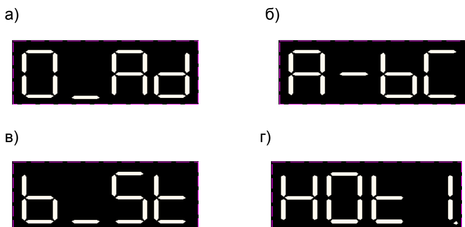
Рисунок 3 – Индикация сигналов замыкания ( 3а ) и обрыва ( 3б ) платиновых ТС, например, канала А
