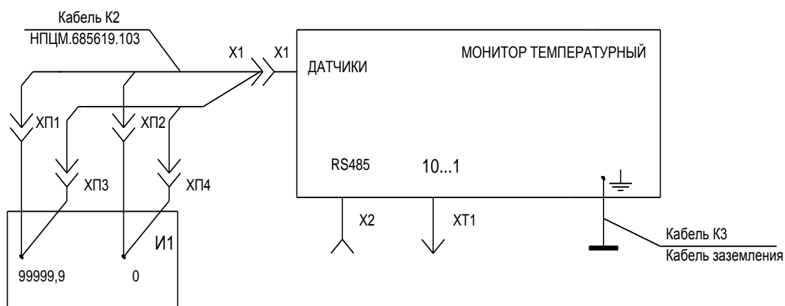
Рисунок 5 – Схема проверки прибора
