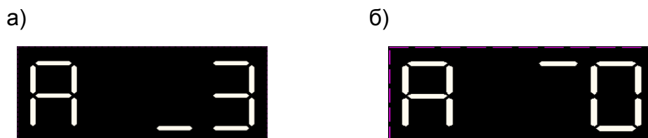
Рисунок 3 – Индикация сигналов замыкания ( 3а ) и обрыва ( 3б ) платиновых ТС, например, канала А
