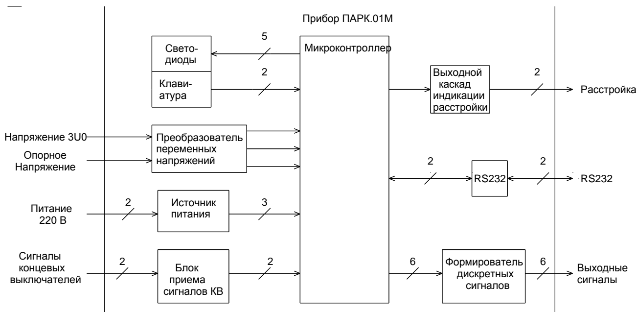
Рисунок 1 – Структурная схема прибора
