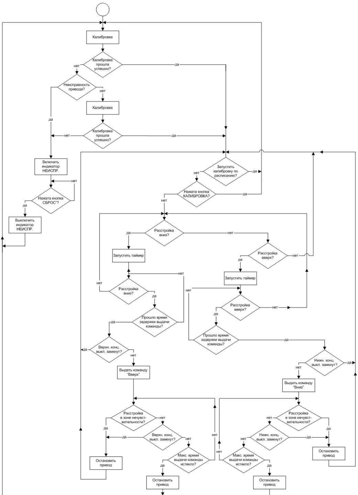
Рисунок Б.1 - Схема алгоритма регулирования прибора
