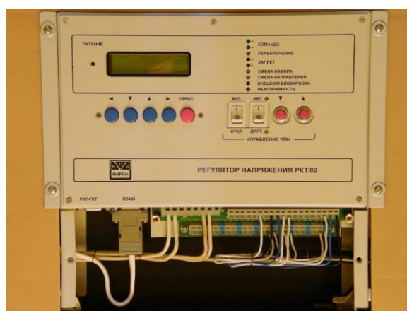
Рис3: Вид монтажа
